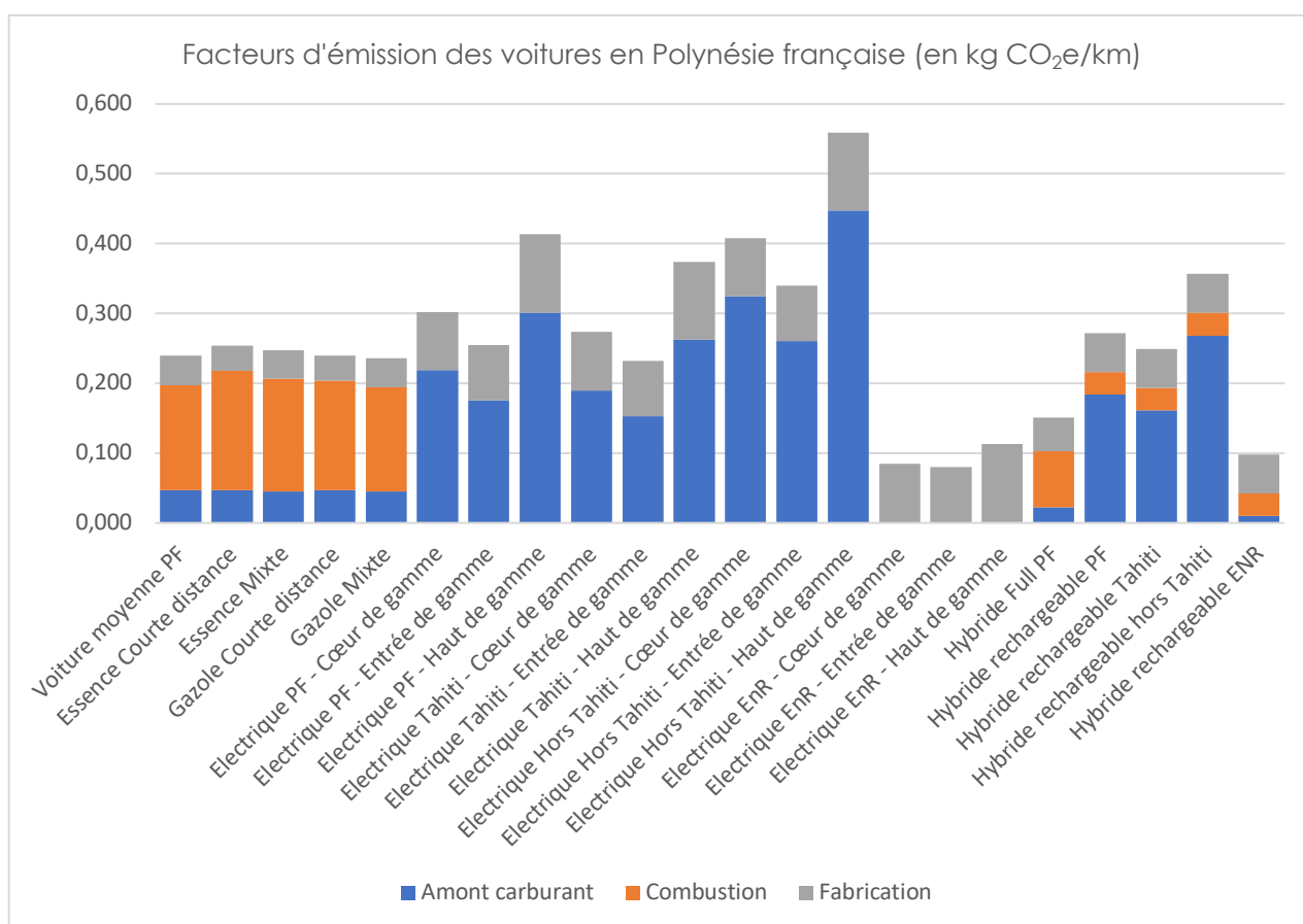
Figure 3 : Facteurs d'émission des voitures en Polynésie française (en kg CO 2 e/km)
